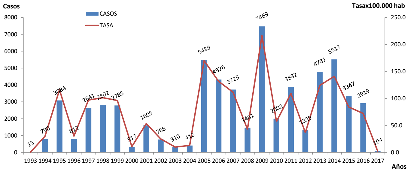
Gráfico Nº 1 Número de casos de dengue y tasa de incidencia según año de ocurrencia en la República de Panamá-período 1993-2017 (sem 3)
